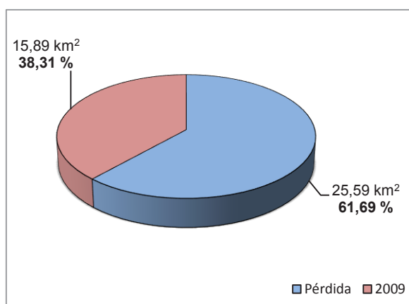
Gráfico 21. Pérdida de superficie glaciár entre 1970 y 2009 en la cordillera Urubamba
