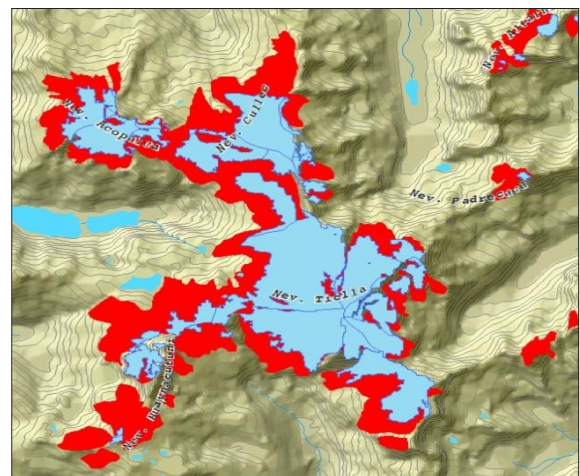
Figura 17. Reducción de la superficie glaciar 1970 y 2007 vista en los nevados Tielia y Cullec.
