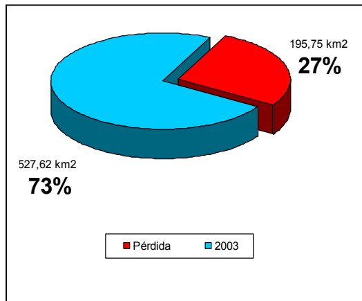
Gráfico 3. Píndida de cobertura glaciaria entre 1970 y 2003 de la cordillera Blanca.
