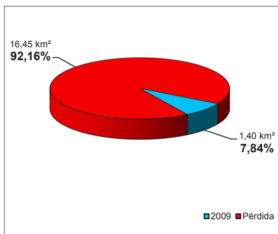
Gráfico 14. Pérdida de superficie glaciar entre 1970 y 2009 en la cordillera Chonta.
