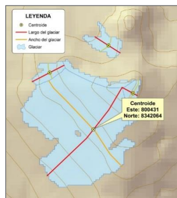
Figura 4. Centroides de un glaciar.
