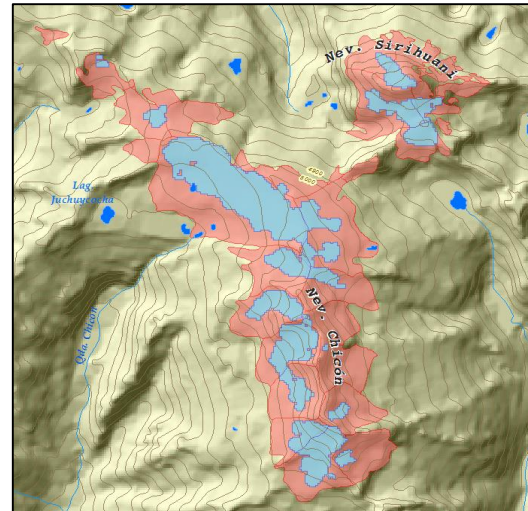
Figura 30. Retracción y desaparición de glaciares de montaña en la cordillera Urubamba.
