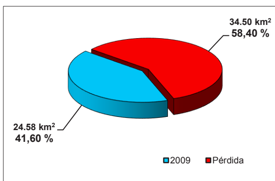
Gráfico 12. Pérdida de superficie glaciaria entre 1970 y 2009 en la cordillera Huaytapallana.
