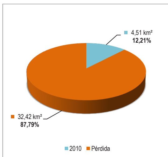
Gráfico 23. Pérdida de superficie glaciar entre 1970 y 2010 en la cordillera Huanzo.
