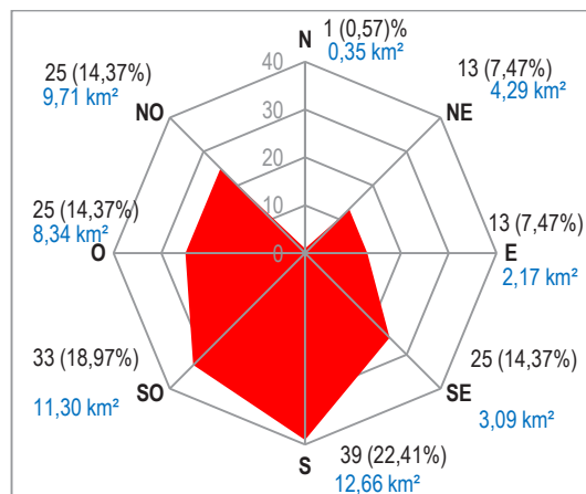
Gráfico 7. Orientación de los glaciares según rango de tamaño
