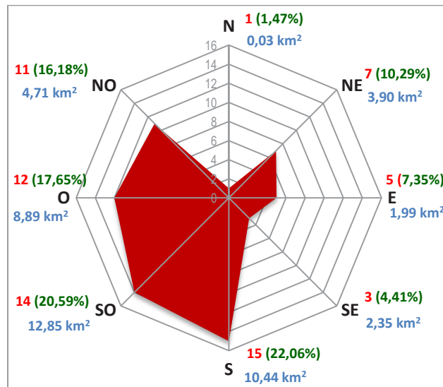
Gráfico 32. Orientación de los glaciares según rango de tamaño
