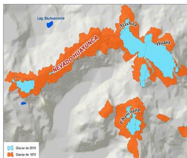
Figura 31. Reducción de la superficie glaciar entre 1970 y 2010 en el Nevado Huayunca.
