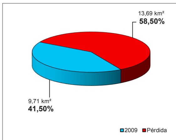
Gráfico 10. Pérdida de superficie glaciar entre 1970 y 2009 en la cordillera Huagoruncho.
