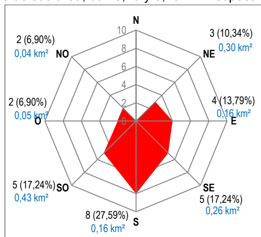
Gráfico 13. Orientación de los glaciares según rango de tamaño.
