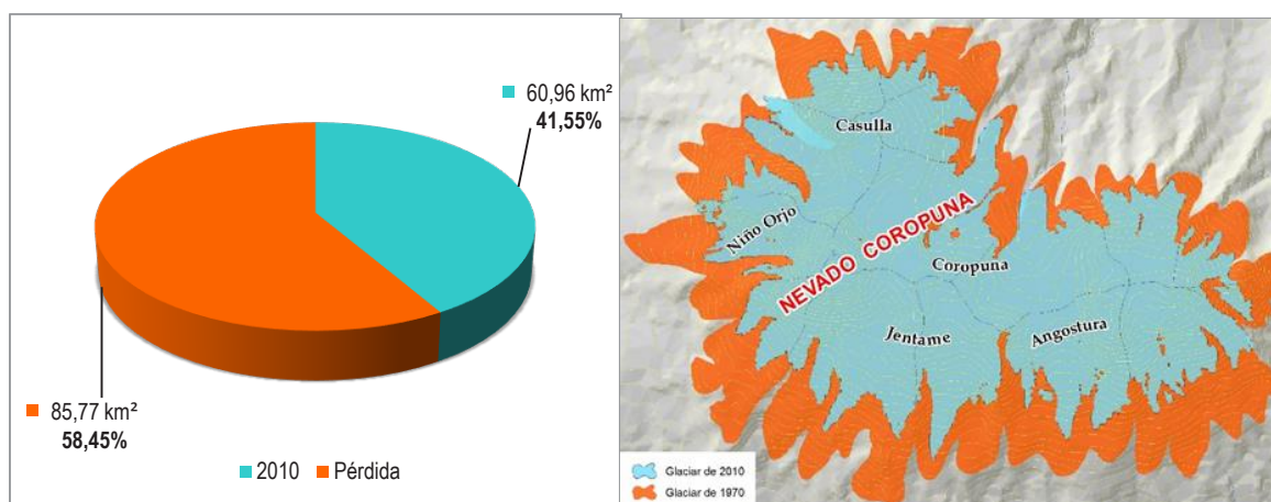
Gráfico 16. Pérdida de superficie glaciar entre 1970 y 2010 en la cordillera Ampato.
