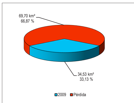
Gráfico 31. Pérdida de superficie glaciar entre 1970 y 2009 en la cordillera Carabaya.
