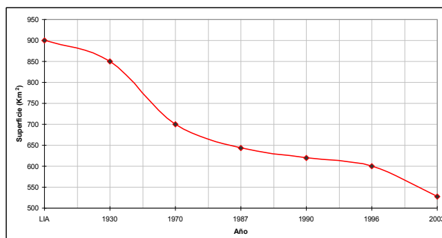
Gráfico 2. Fluctuación de la cobertura glaciar en la Cordillera Blanca desde el fin de la Pequeña Edad de Hielo.
