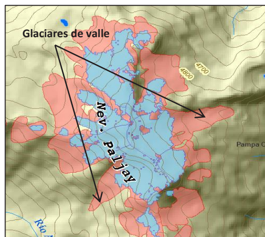
Figura 28. Retracción de un glaciar de valle a un glaciar de montaña en la cordillera Vilcabamba.
