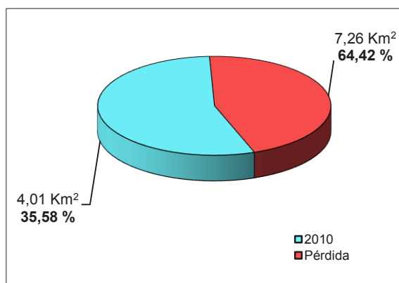
Gráfico 27. Pérdida de superficie glaciar entre 1970 y 2010 en la cordillera La Raya.
