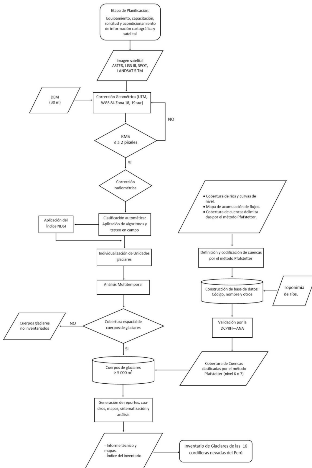
Diagrama 1. Metodología del inventario de glaciares.
