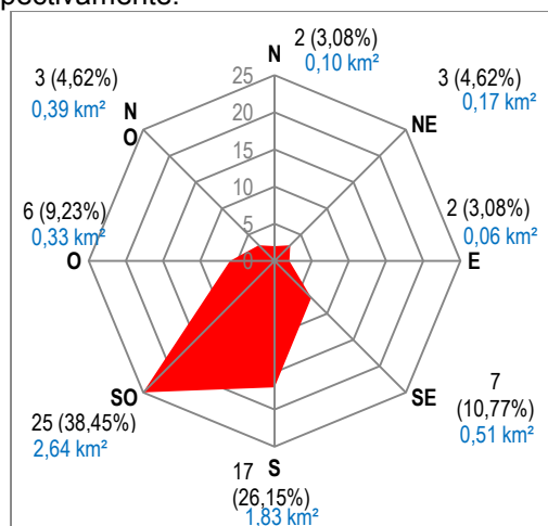
Gráfico 5. Orientación de los glaciares según rango de tamaño.
